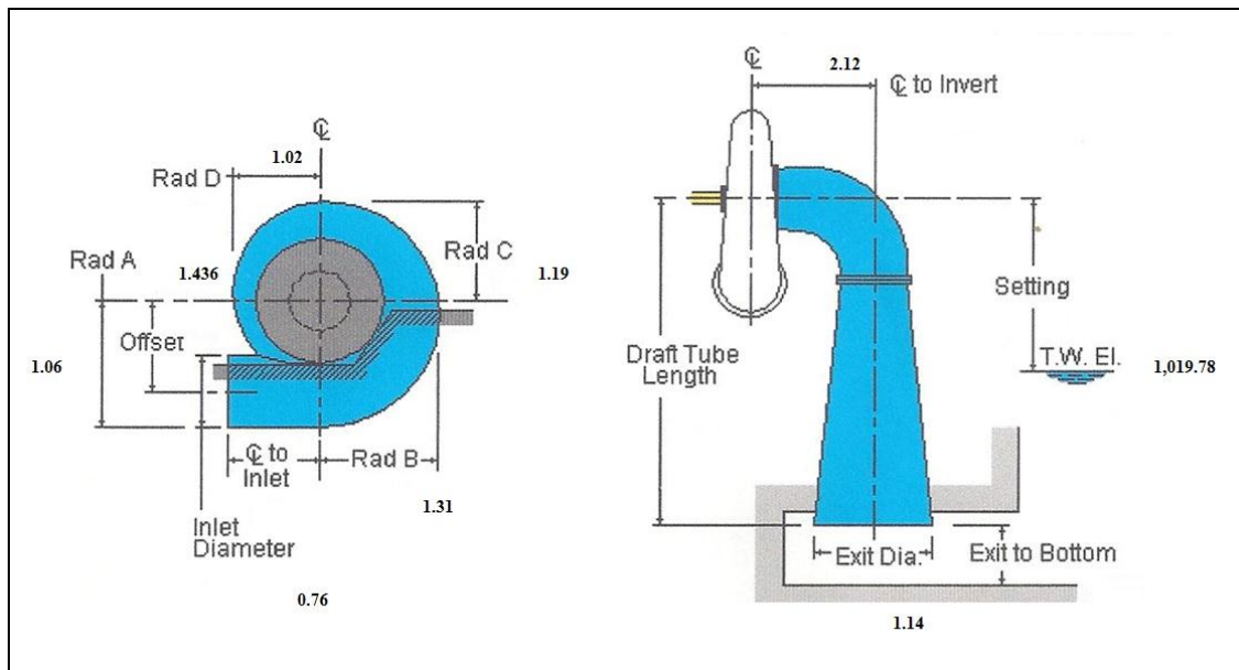
Imagen 2.15. Dimensiones preliminares para turbina de 4 m 3 /s
