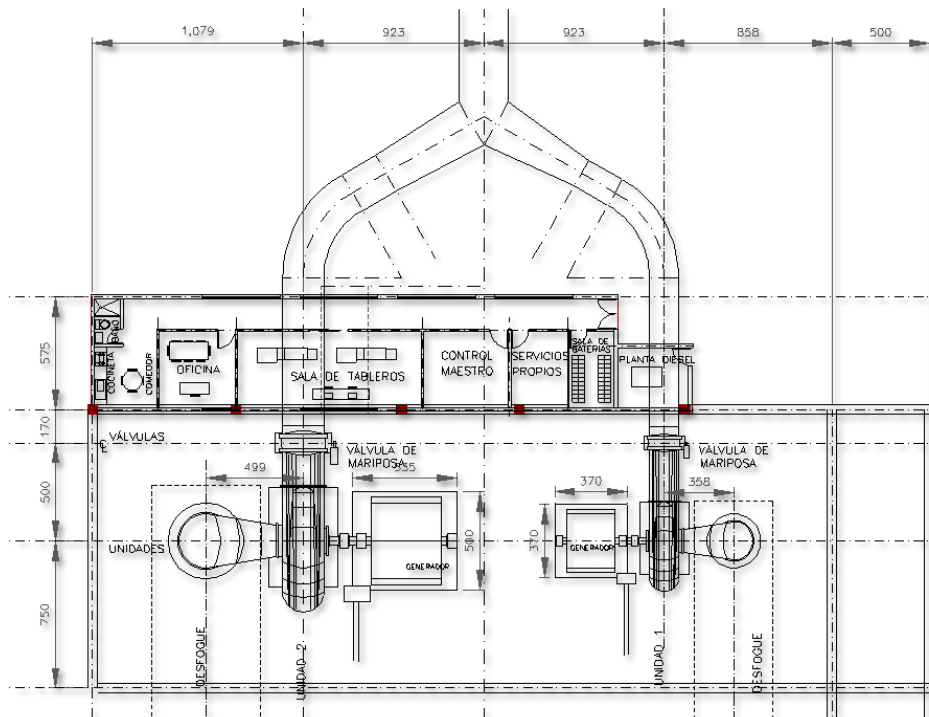
Imagen 2.16. CM, vista en planta
