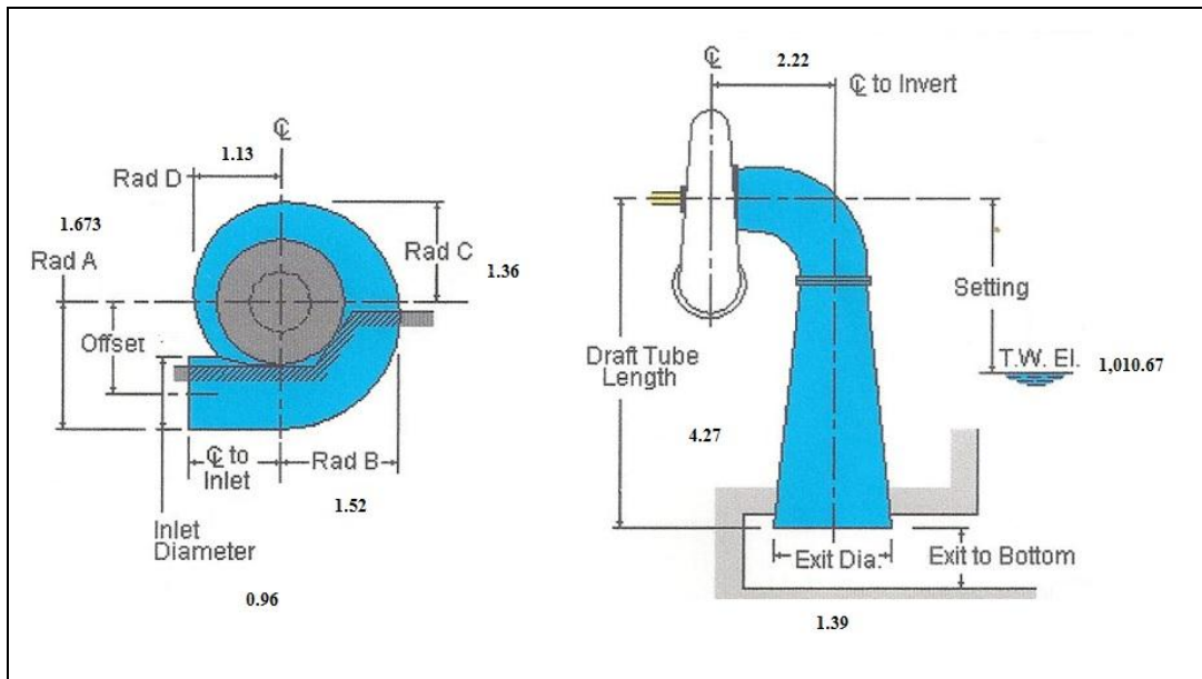
Imagen 2.14. Dimensiones preliminares para turbina de 8 m 3 /s.
