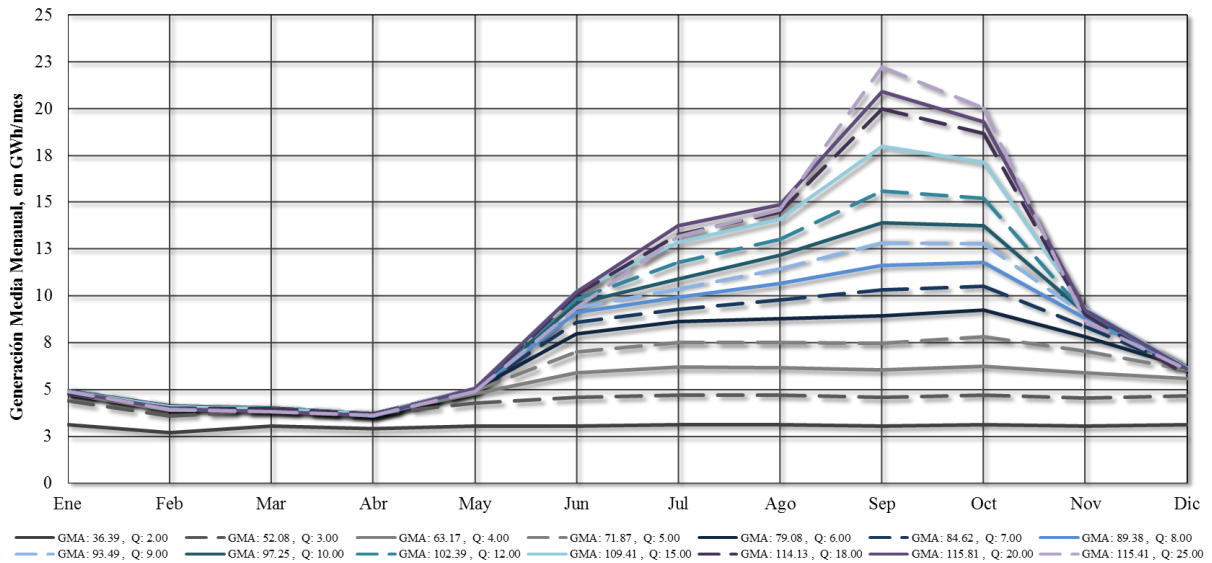
Gráfica 2. 6. Curvas de generación media mensual para diferentes gastos de equipamiento.
