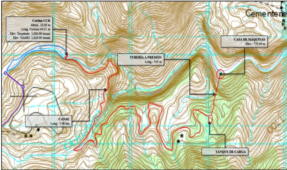
Imagen 2.4. Esquema de obras para el proyecto.
