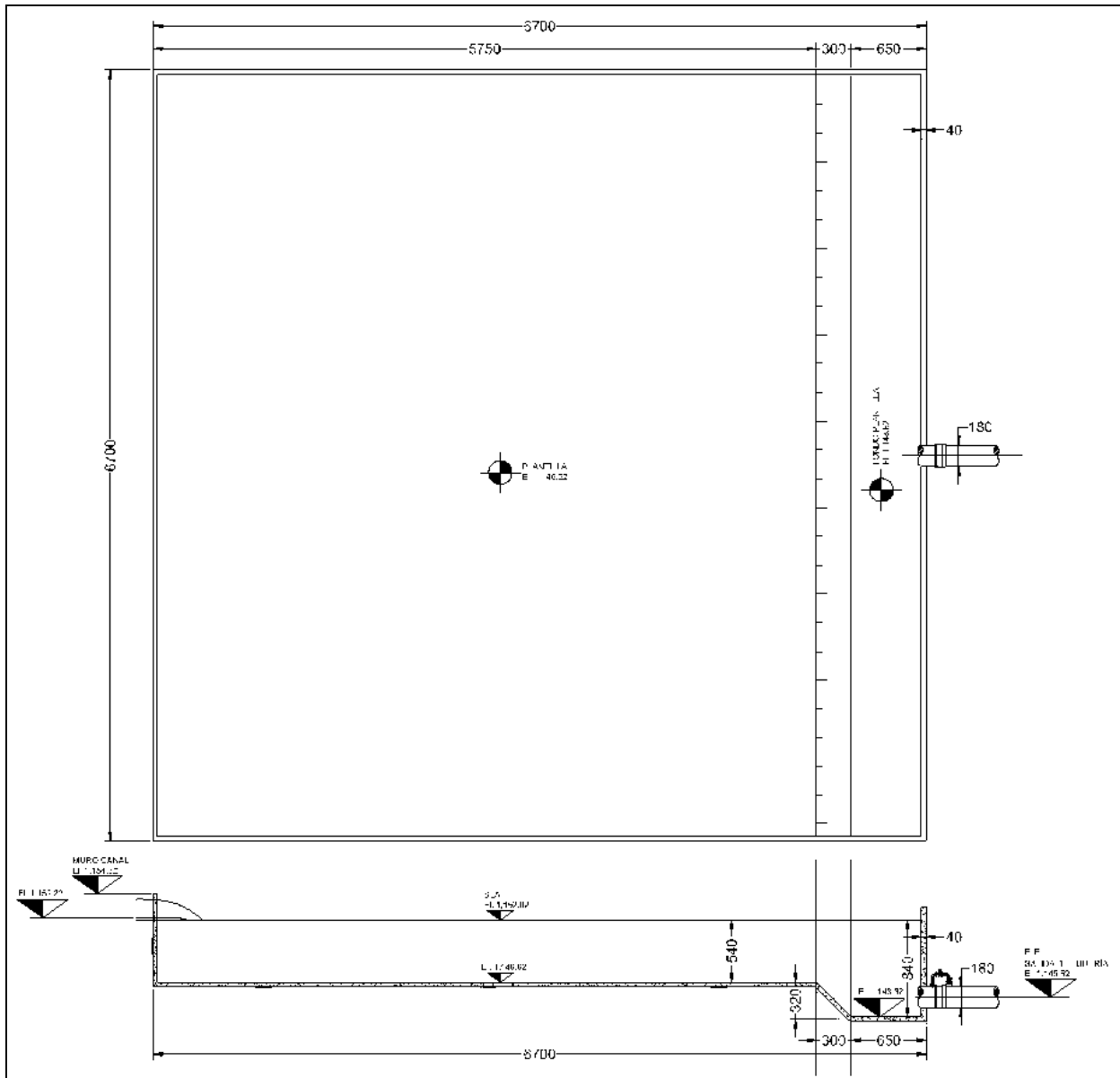
Imagen 2.12. Vista en planta del TR. Dimensiones en cm.
