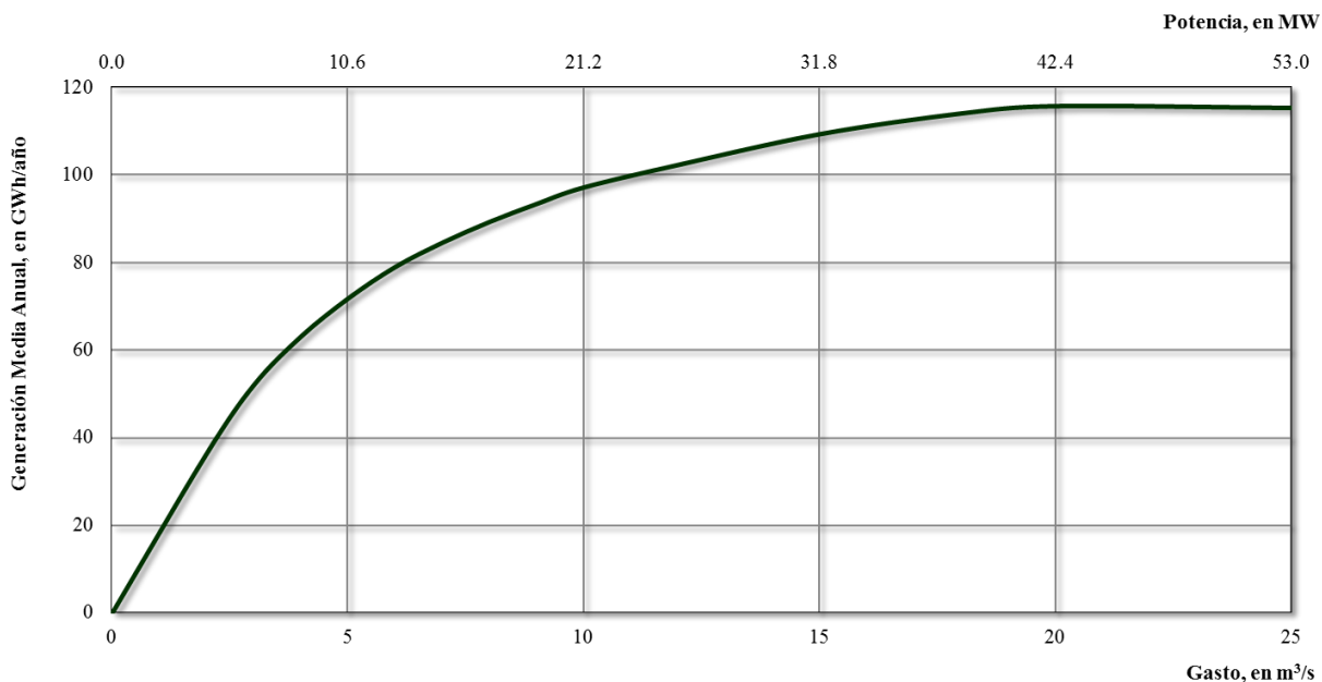
Gráfica 2.5. Curva de generación media anual, para dos unidades.
