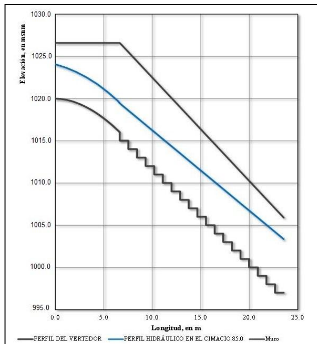
Gráfica 2.8. Perfil hidráulico en rápida escalonada.
