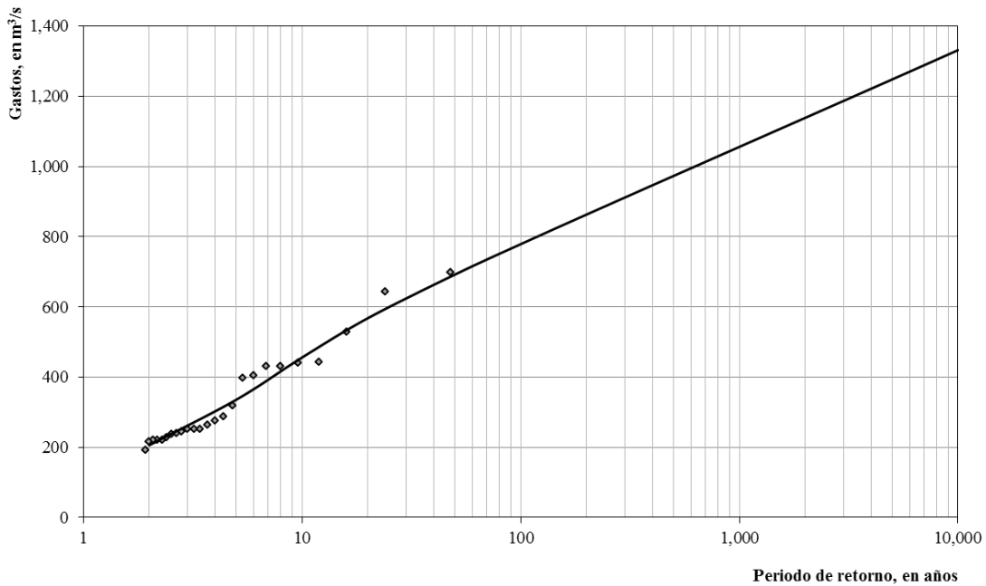
Gráfica 2.4. Avenidas de diseño para el proyecto.
