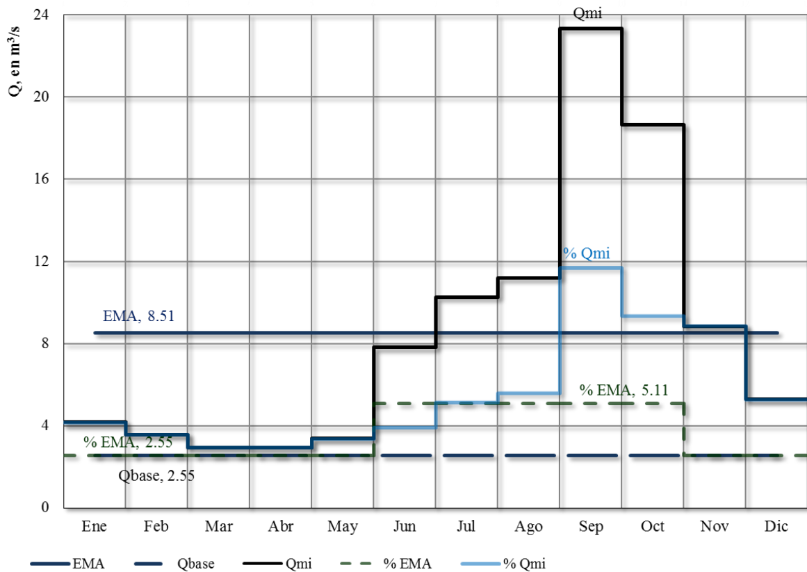
Gráfica 2.2. Gastos medios mensuales en la captación del proyecto, en el Río Apulco
