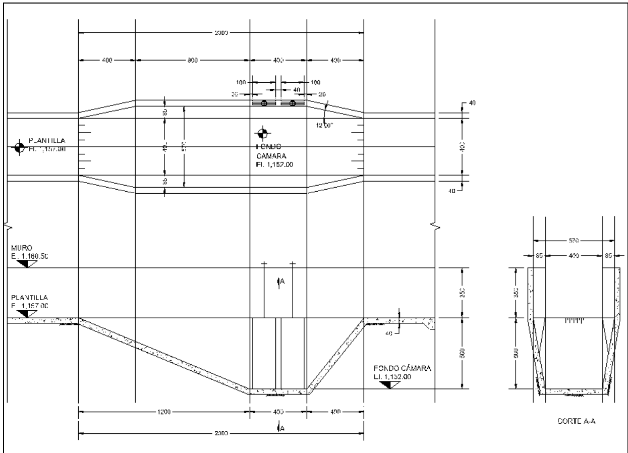
Imagen 2.9. Dimensiones del desarenador.
