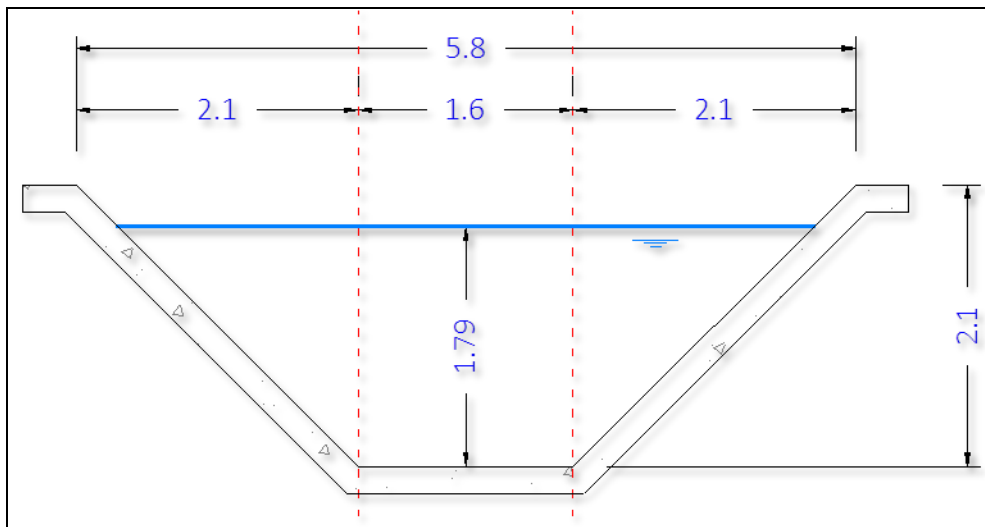
Imagen 2.10. Sección transversal del canal de conducción, para un caudal de 12 m 3 /s
