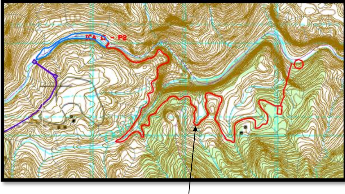
Imagen 2.11. Trazo del Canal de Conducción.
