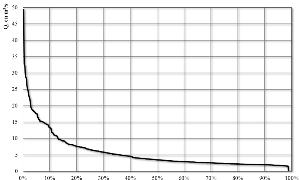
Gráfica 2.3. Curva de Gastos – Probabilidades en la zona de captación del proyecto, en el Río Apulco
