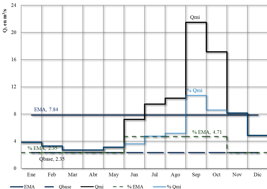
Gráfica 4.4. Gastos medios mensuales en la captación del proyecto, en el río Apulco
