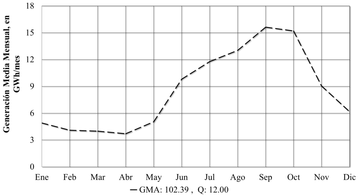
Gráfica 2. 7. Generación media mensual para un gasto de equipamiento de 12 m 3 /s, para el proyecto.
