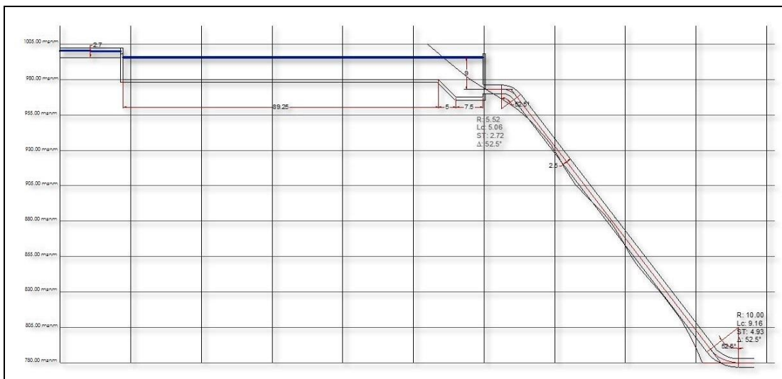
Imagen 2.13. Perfil de TP para gasto de 12 m 3 /s
