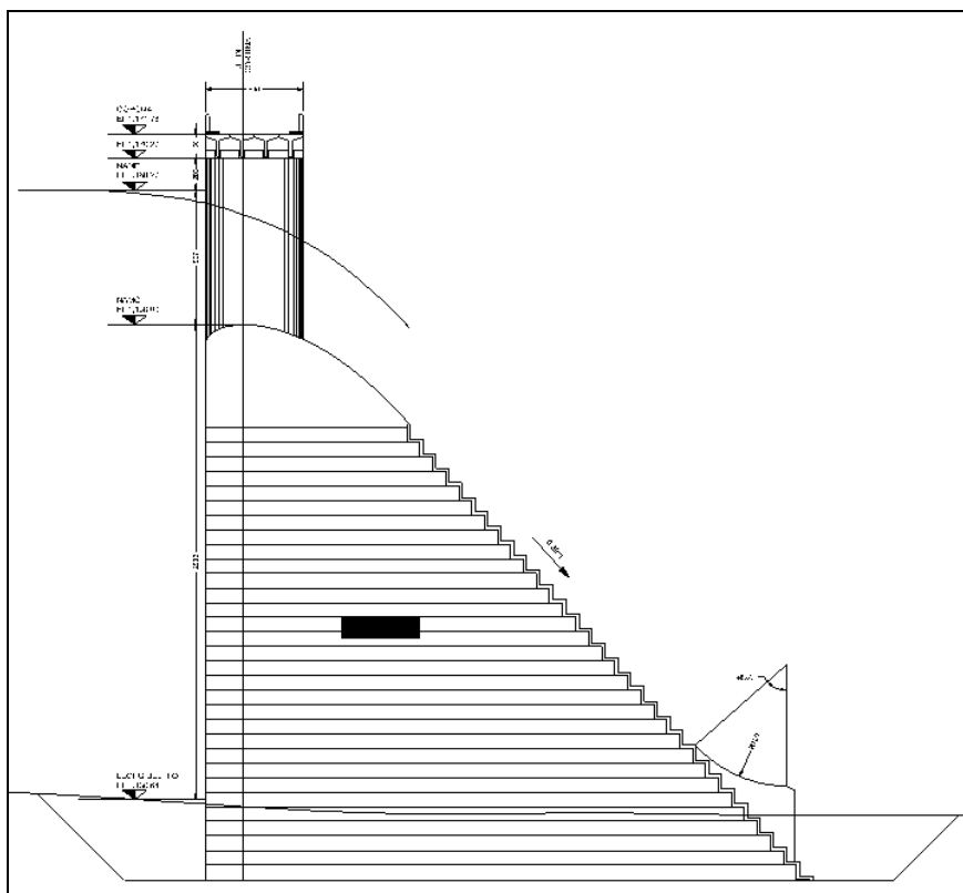
Imagen 2.7. Obra de Contención.
