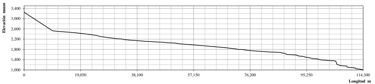
Gráfica 4.1. Perfil del cauce principal de la cuenca de aportación para el proyecto.
