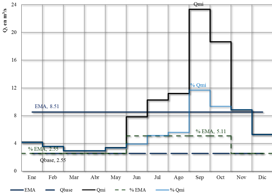
Gráfica 2.1. Estimación de caudal ecológico para el proyecto.
