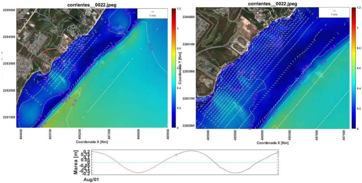
Figura 6-37. Corrientes generadas durante la llenante.
