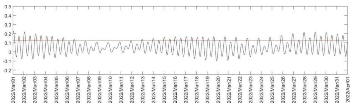
Figura 6-18. Representación gráfica de la marea para el mes de marzo de 2022 en donde se aprecia el régimen de marea caracterizado como semidiurna
