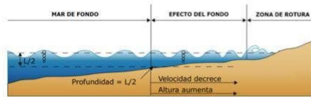
Figura 6-23. Esquema de la rotura del oleaje por fondo. La profundidad disminuye causando que la velocidad decrezca, la altura de la ola aumente y rompa con la consecuente pérdida de energía.
