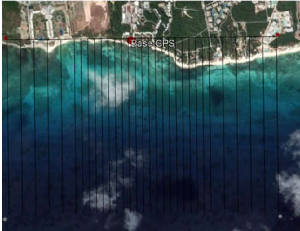
Área del levantamiento batimétrico y transectos planificados
