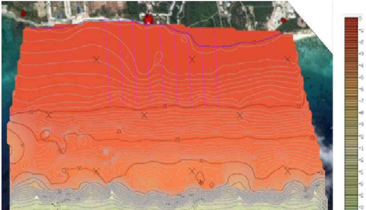
Figura 6-8. Mapa de curvas de nivel de profundidades (isobatas).
