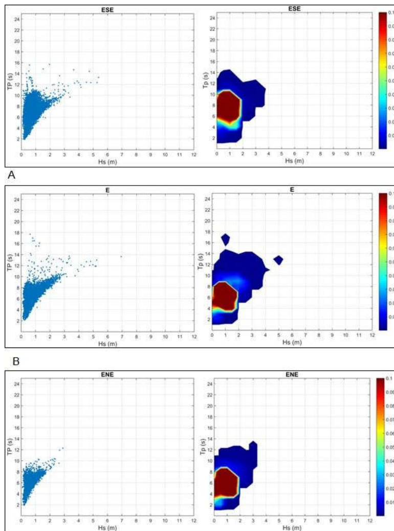
Figura 6-14. Frecuencia de ocurrencia conjunta Hs-Tp, para oleaje en aguas profundas
