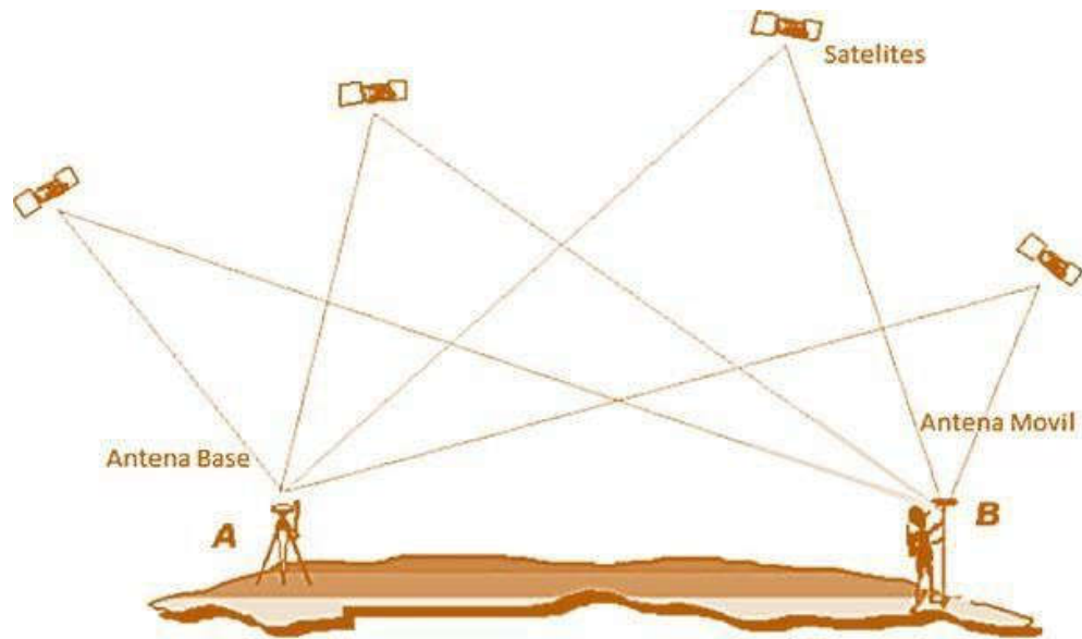
Figura 6-1. Esquema de componentes que conforman el sistema GNSS diferencial
