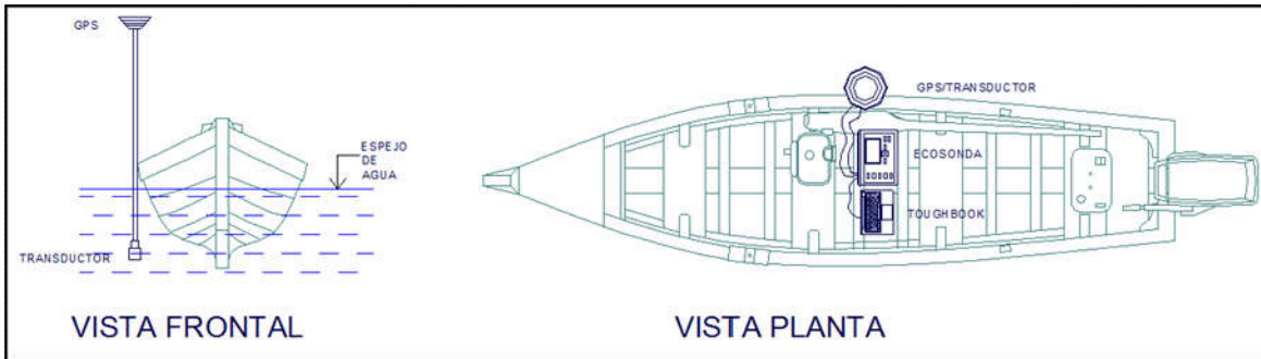
Figura 6-6. Esquema de colocación de equipos
