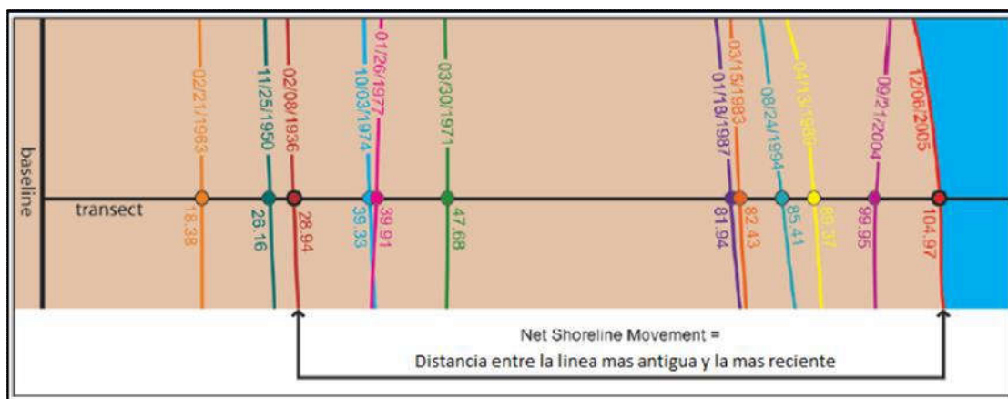
Figura 6-31. Ejemplo de NSM entre dos líneas de costa
