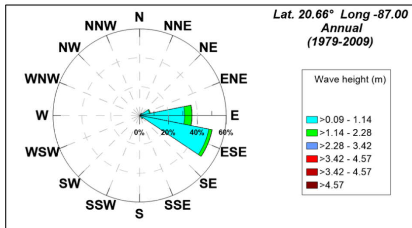
Rosa de oleajes respecto a la magnitud de H_s
