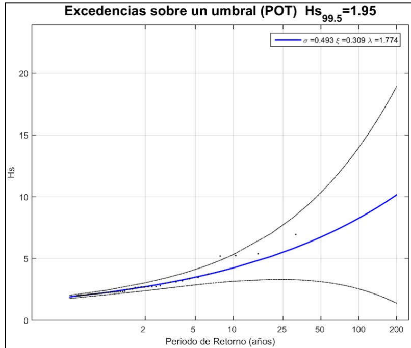
Figura 6-15. Régimen extremal escalar de altura de ola ( H_s ).
