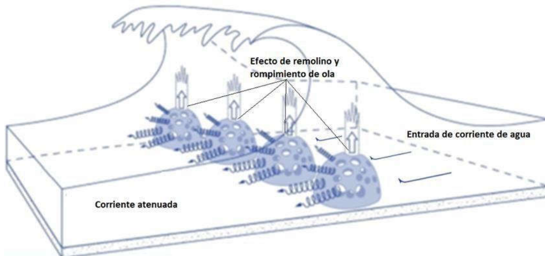
Figura 6-39. Esquema de disipación de energía de oleaje por efecto de Reef-Ball™
