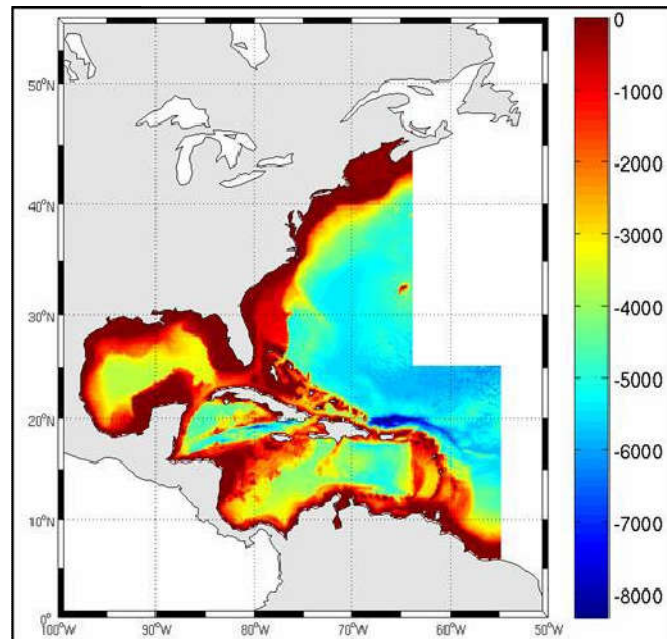
Figura 6-11. Batimetría utilizada para el Golfo de México y el Atlántico Noroeste, nodos a cada 10 minutos.
