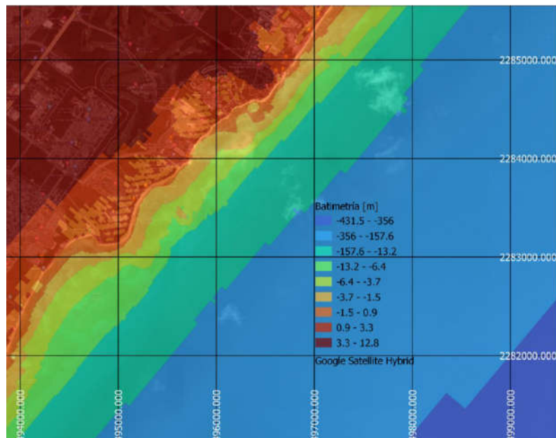
Batimetría de la zona de estudio para malla global
