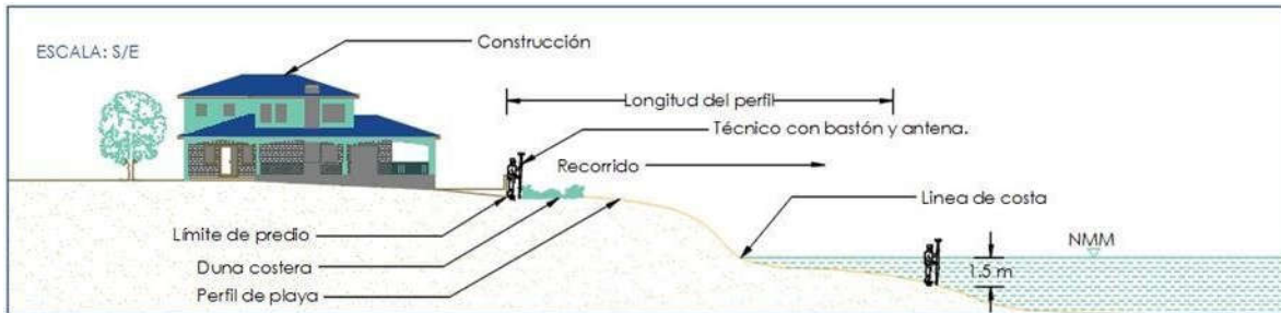
Figura 6-3. Recorrido tipo de levantamiento de perfiles de playa
