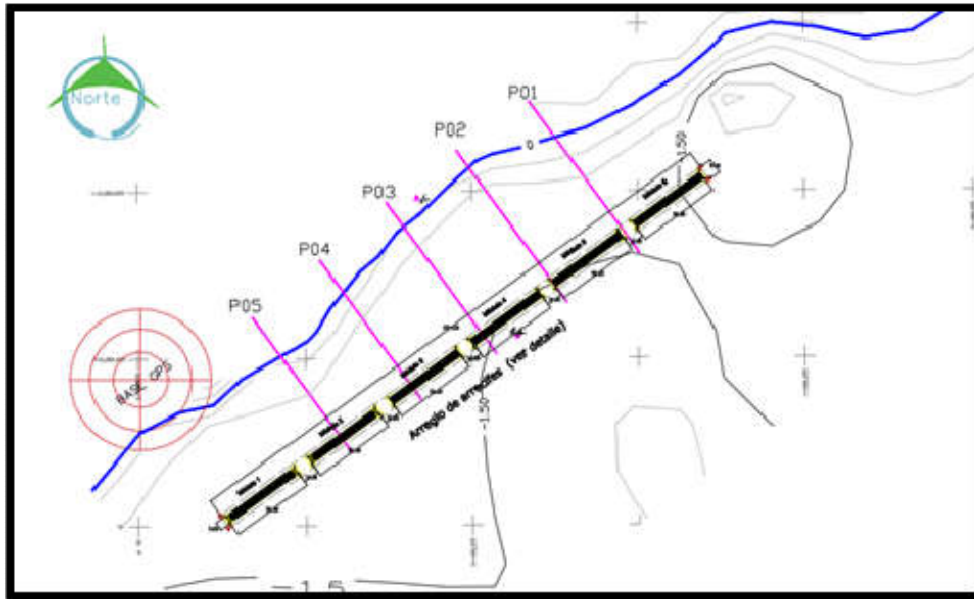
Planta general de ubicación de arrecifes artificiales.
