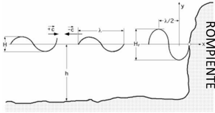
Figura 6-21. Reflexión de una ola. Las olas se reflejan en la barrera disminuyendo o anulando los movimientos horizontales de las partículas debido a las ondas incidentes y reflejadas.
