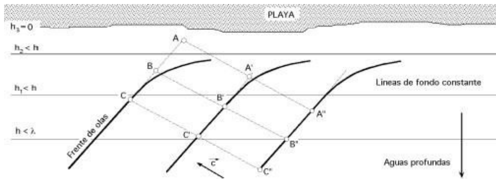
Figura 6-20 Refracción de un tren de olas. La ola se afecta cuando la profundidad del agua es igual a la mitad de su longitud de onda ( h = \lambda/2 ) y afecta su frente de propagación al acercarse a la playa.
