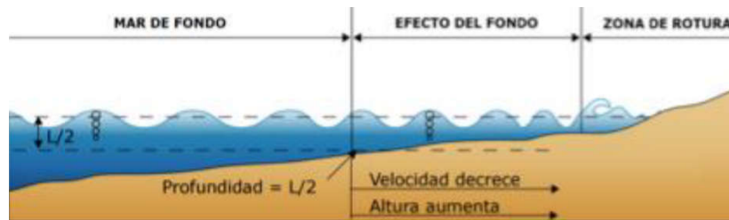
Esquema de la rotura del oleaje por fondo. La profundidad disminuye causando que la velocidad decrezca, la altura de lo ola aumente y rompo con lo consecuente pérdida de energía.
