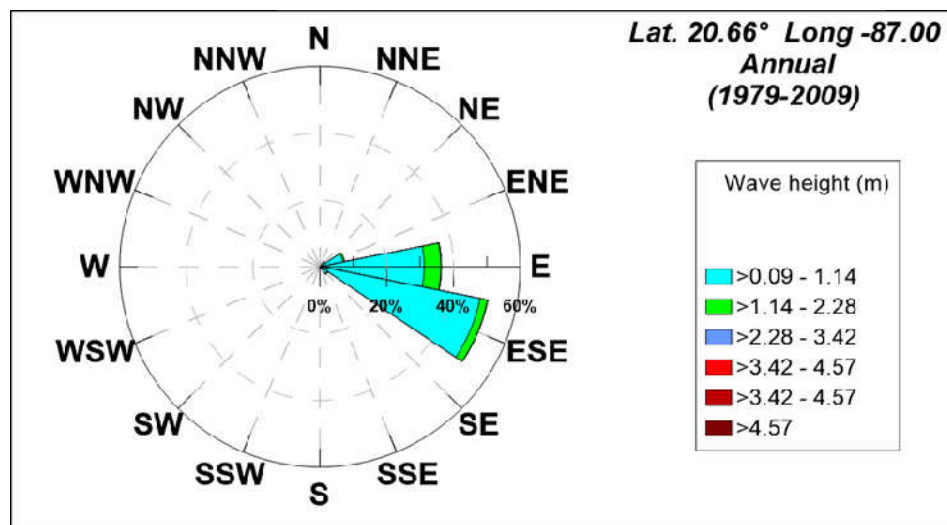
Figura 6-13. Rosa de oleajes medios respecto a la magnitud de Hs.
