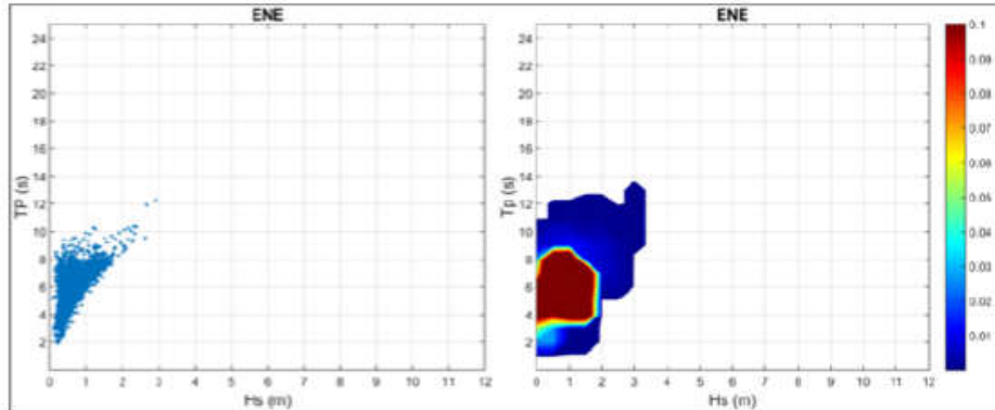
Frecuencia de ocurrencia conjunta Hs-Tp para oleaje en aguas profunda
