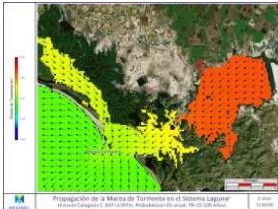
Propagación de la onda de marea de tormenta en el sistema lagunar Santa María-Topolobampo-Ohuira. Caso de estudio huracán categoría 5 a las 12:00 horas de iniciado el evento.
