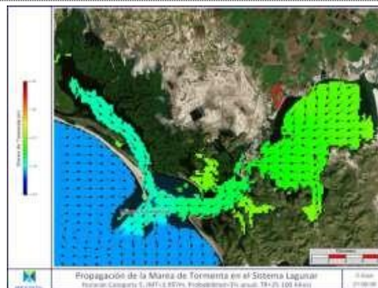
Propagación de la onda de marea de tormenta en el sistema lagunar Santa María-Topolobampo-Ohuira. Caso de estudio huracán categoría 5 a las 21:00 horas de iniciado el evento.
