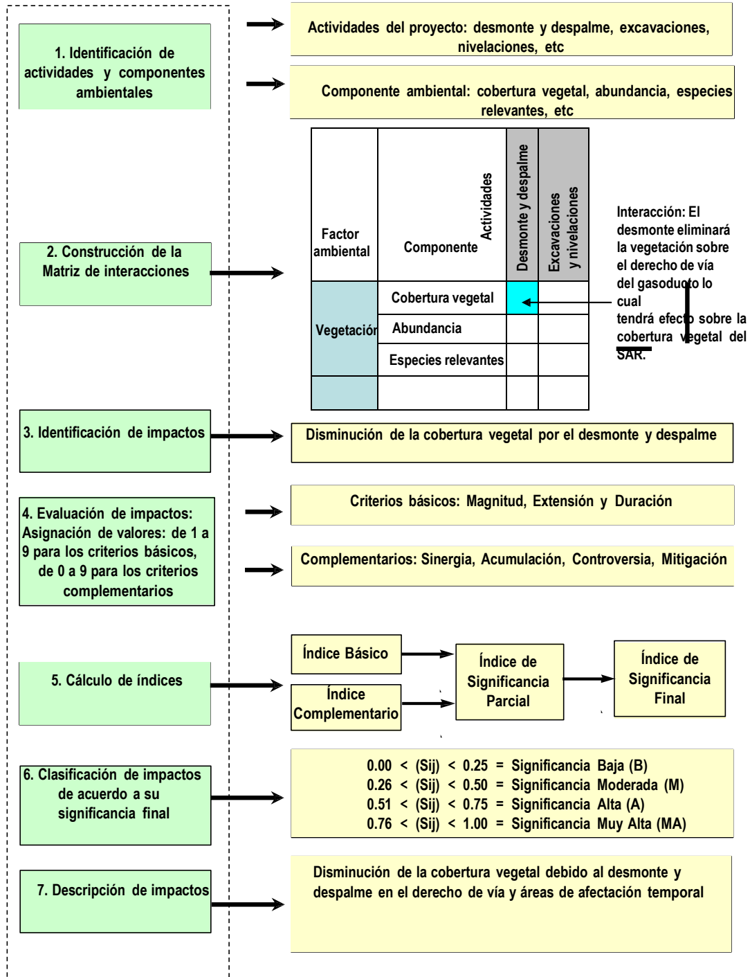
Figura 1. Esquema metodológico.
