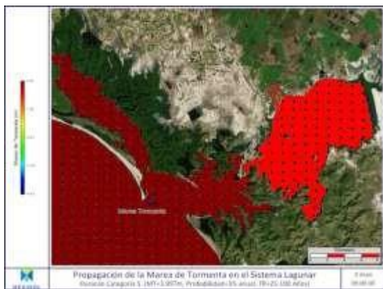
Propagación de la onda de marea de tormenta en el sistema lagunar Santa María-Topolobampo-Ohuira. Caso de estudio huracán categoría 5 a las 06:00 horas de iniciado el evento
