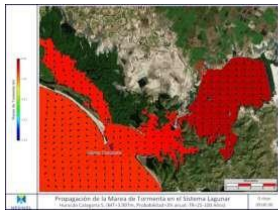
Propagación de la onda de marea de tormenta en el sistema lagunar Santa María-Topolobampo-Ohuira. Caso de estudio huracán categoría 5 a las 09:00 horas de iniciado el evento
