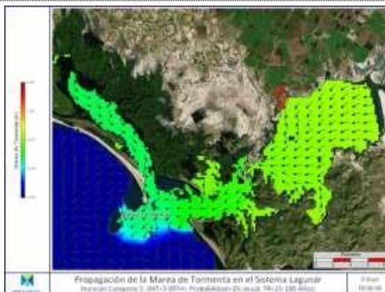
Propagación de la onda de marea de tormenta en el sistema lagunar Santa María-Topolobampo-Ohuira. Caso de estudio huracán categoría 5 a las 18:00 horas de iniciado el evento
