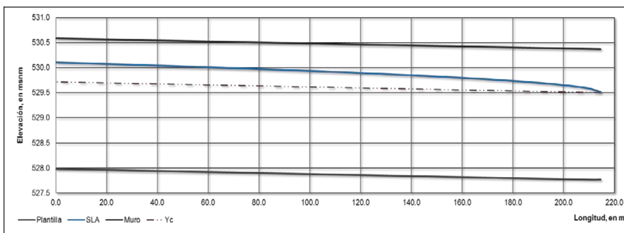
Figura II.12. Perfil hidráulico en el canal de conducción
