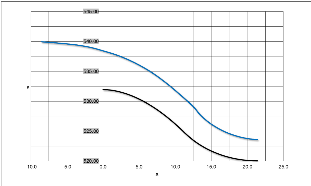
Figura II.17. Perfil hidráulico en vertedor.
