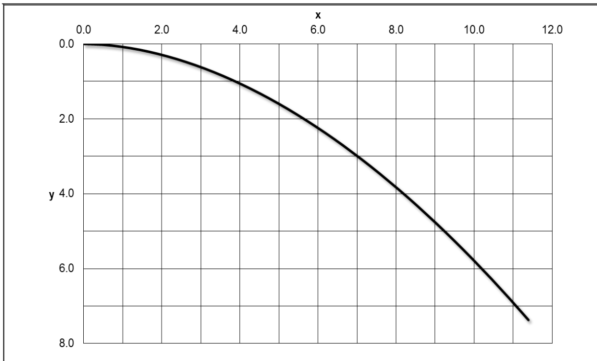
Figura II.16. Perfil del cimacio, paramento de aguas arriba vertical
