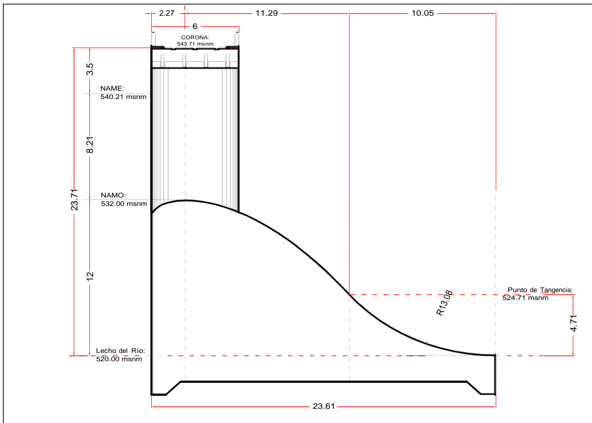
Figura II.12. Obra de Contención, corte por sección vertedora
