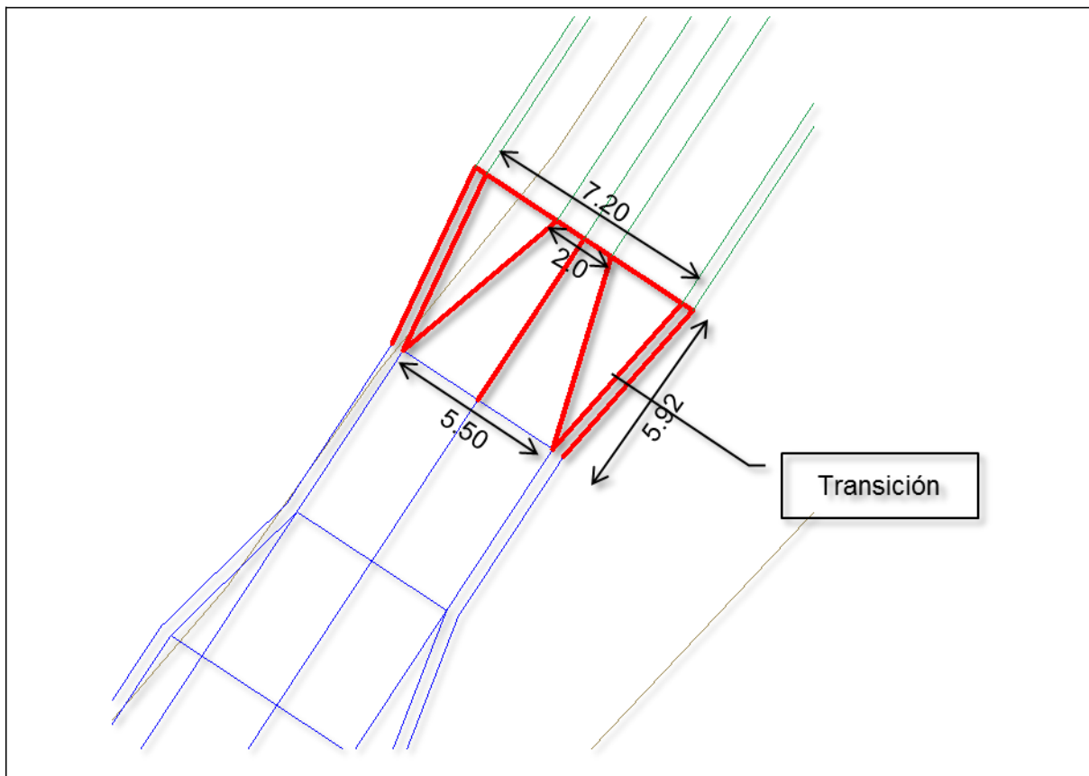
Figura II.13. Transición Sección Trapecial – Rectangular
