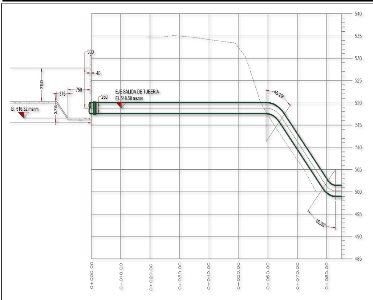
Figura II.15. Perfil de tubería a presión para gasto de 22m 3 /s
