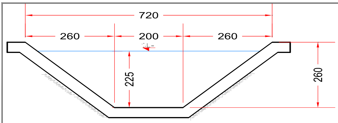
Figura II.11. Sección transversal del canal de conducción
