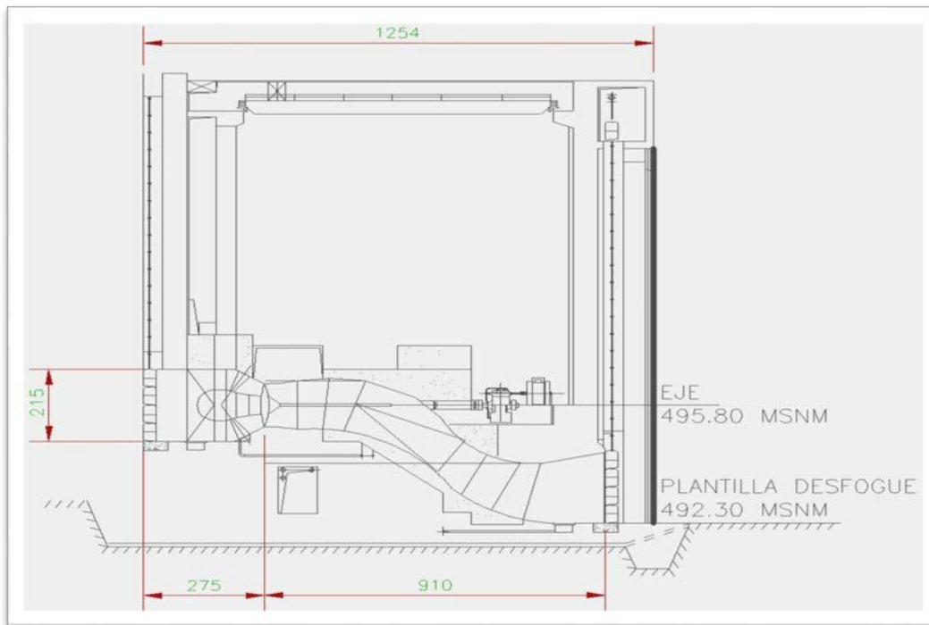
Figura II.25. Casa de máquinas, Corte por unidad 1
