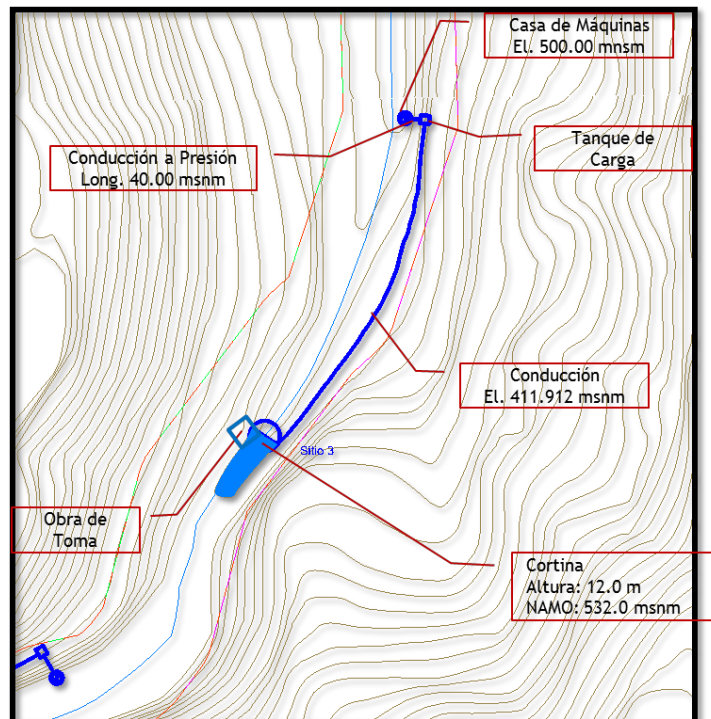
Figura II.10. Cartografía topográfica de localización de la obra de toma hasta la casa de máquinas del proyecto MHE “Virgen de Guadalupe”
